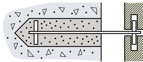
Fig 3.6 Hällarkramla av plattstång, ingjuten i betongstomme.
