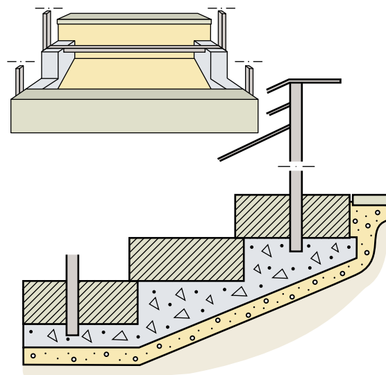
Fig 7.30 Räcke monterat i ett infästningsstål under blockstegen, som är monterade på längsgående balkar.
