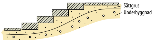
Fig 7.19 Montering av blocksteg på underbyggnad av grus eller samkross
