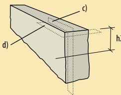
c) Vinkelräthet mellan översida och fogsida intill måttet h2. d) Vinkelräthet mellan framsidans och fogsidans övre kantlinjer.
