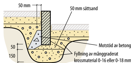
Fig 6.17 Typkonstruktion KG
