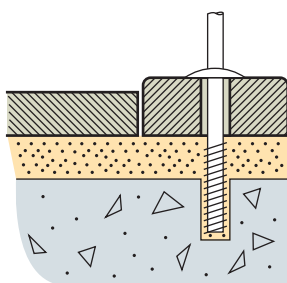
Fig 5.34 Infästning av räcke genom skurlist.
