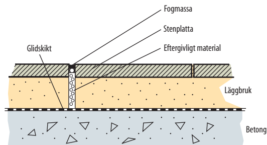
Fig 4.31 Vid fortsatt lagging avlägsnas mothållet och eftergivligt material, t.ex. remsa av cellplast, läggs in för avdelning av läggbruket.
