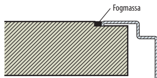
Fig 8.9 Planmonterad ho och häll
