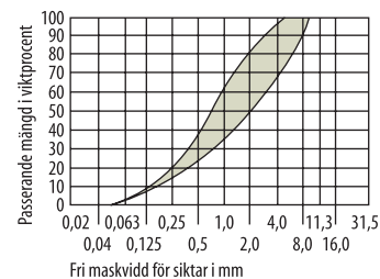
Fig 3.1 Ideala siktkurvor för naturlig sand till läggbruk (enl. Hus AMA 98). Den övre kurvan gäller för tunna skikt och den nedre för tjockare.
