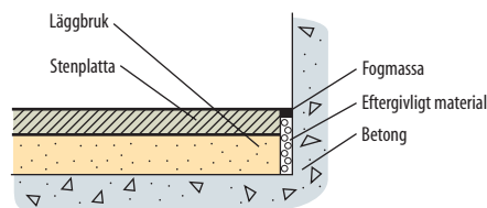
Fig 4.36 När inte fogen täcks av sockel fogas den med elastisk fogmassa.
