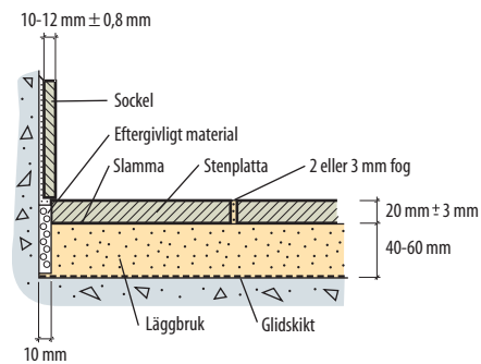
Fig 4.17 Läggningskonstruktion G1.
