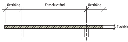
Fig 8.13 Konsolavstånd, överhäng och stentjocklek.
