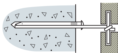
Fig 6.16 Hållarkramla typ HIT 2. Kramla av Ø2 mm rostfri, hård tråd som monteras i Ø5-6 mm hål i betongvägg och låses med rostfri eller galvaniserad spik. Hål, tråd och spik avpassas så att spiken "drar" när den slås in i hålet. Tråden viks runt Ø3 mm dubb som monteras i hål i plattkanterna.
