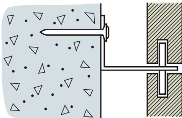
Fig 6.14 Hållarkramla typ HIL, vinkelbockad. Hållarkramla av 1-2 mm rostfri plattstång alt vinkelprofil, eller aluminiumprofil med 2-3 mm godstjocklek. Kramlan monteras med skjutspik, spikplugg eller skruv och plugg i bakmur av betong, lättbetong eller tegel. Den kan också monteras i stabilt regelverk eller träunderlag med skruv. En 3-5 mm grov dubb, beroende på plattjocklek och format, går genom kramlan och in i plattkanterna.
