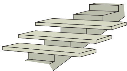
Fig 5.23 Fribärande steg på centralt placerad betongbalk.
