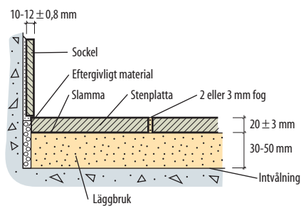
Fig 4.19 Läggningskonstruktion G3.
